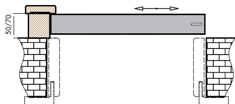
DWUDZIELNE - PRZEKRÓJ POZIOMY
